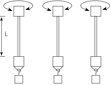
扭转试验说明 固定距离: 0.5m; 扭转角度: \pm 180^\circ 吊重: 500g; 速度: 60 次 / 分钟
